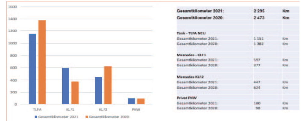
Abbildung 7: Fahrzeugkilometervergleich 2021 / 2020
