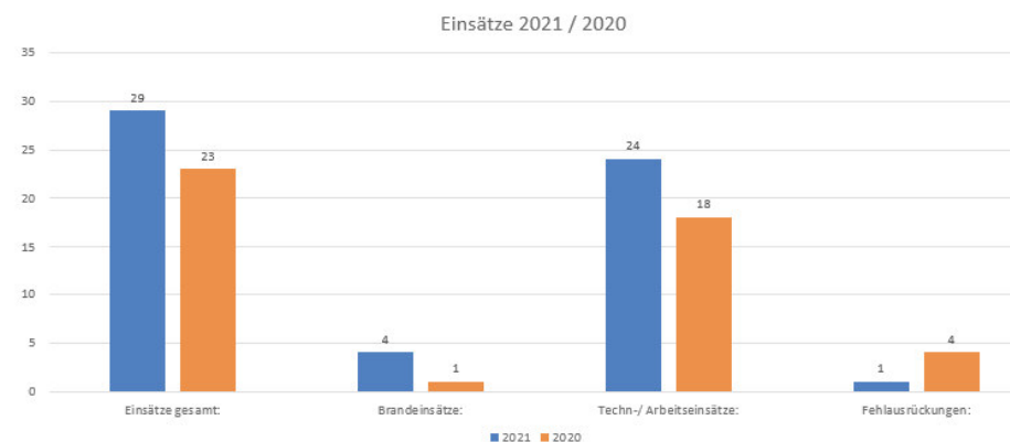
Abbildung 3: Einsatzstatistik
