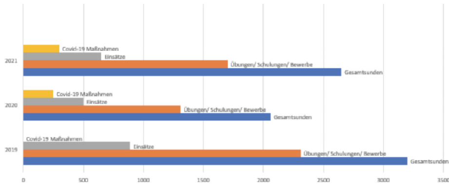
Abbildung 5: Gesamtstundenvergleich 2021/2020/2019
