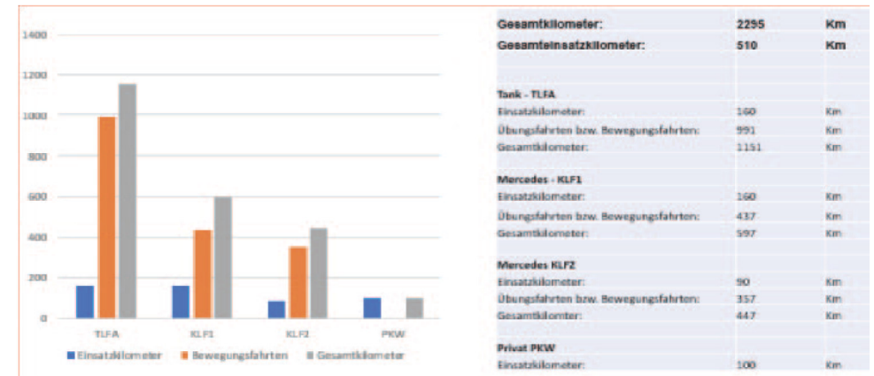
Abbildung 8: Fahrzeugkilometer 2021/2020
